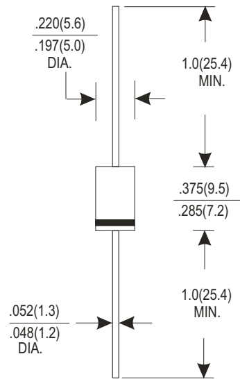
DO-201AD
