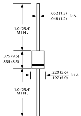
DO-201AD
