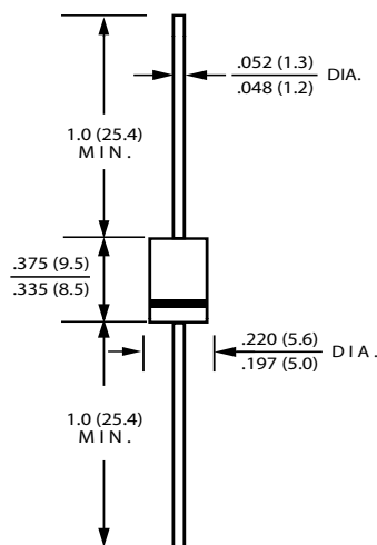
DO-201AD
