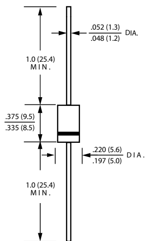
DO-201AD
