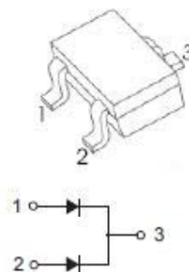
SOT-323
