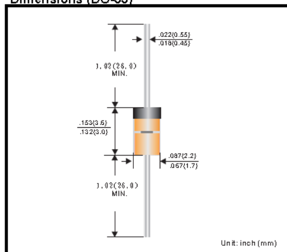
Dimensions (DO-35)
